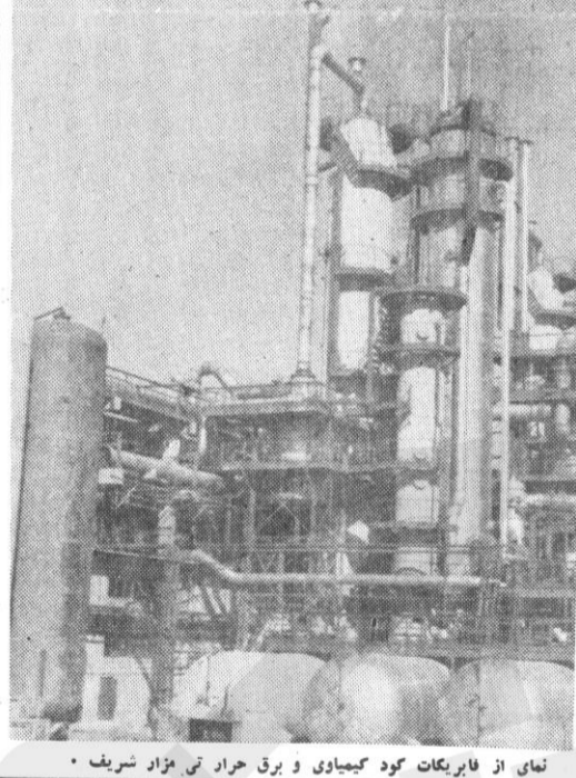
نمای از فابریکات کود کیمیاوی و برق حرارتی مزار شریف.
