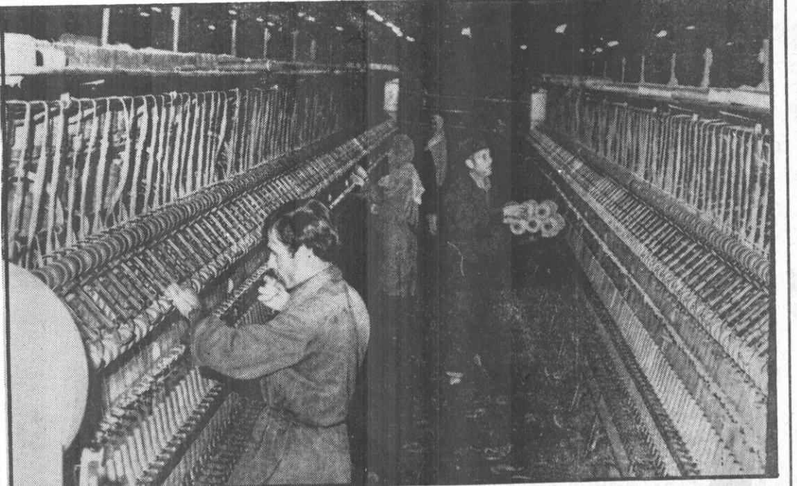
کارگران پشمینه با فسی بلچر خنی این اولین دستگاه صنعتی در رشته صنعت پشمینه بافی کشور، محصولات تولیدی مرغوب و با کیفیت عالی را که نمره کار و توجه زنان و مردان کارگریکه دوشادوش هم وبه شیوه انقلابی در این واحد تولیدی صنعتی کشور مصروف اند، به بازار جهت تامین نیازمندی های هموطنان عرضه میدارند (عکاسی ح.ا.ت)
