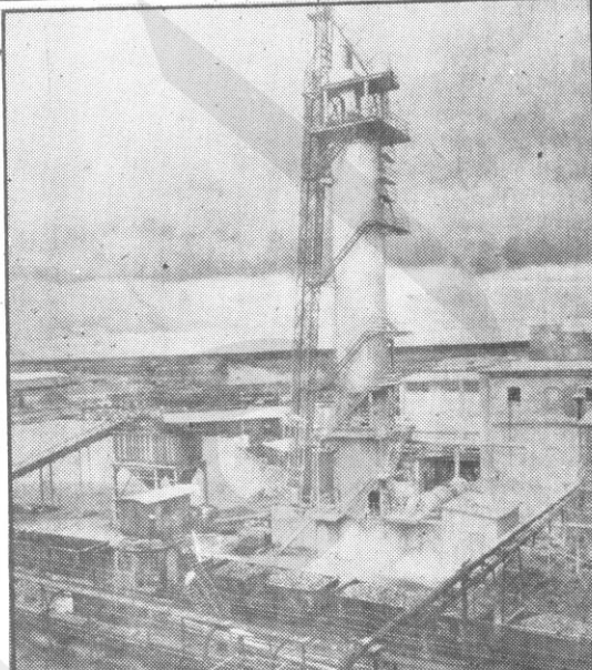
نمای از لایبریکه قند المان دموکراتیک که روزانه ۲۱۰۰ تنه تولید و تصفیه می نماید. برای اولین بار در این لایبریکه تمام مواد تولید آن در فضای آزاد به آب می رسد.
