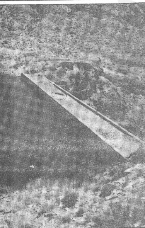
با احیای مجدد بند امیر غازی برای ده هزار جریب زمین زراعتی در بتخاله قنعه محسن، پلچرخ آب تهیه شده است. (عکاسی ح.ا.ث)
