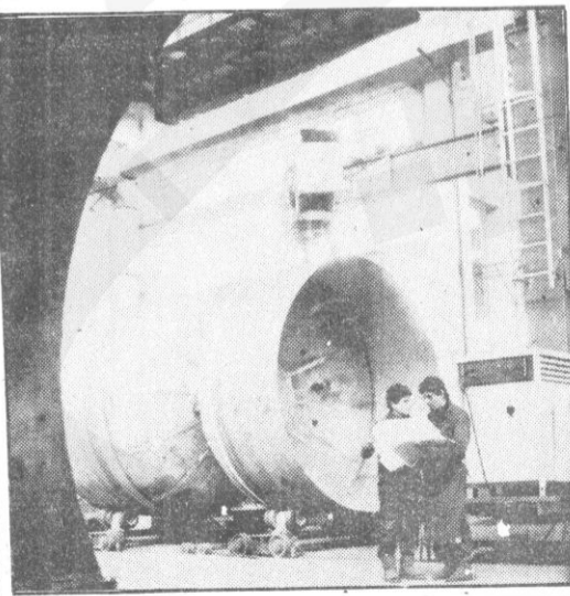
در فابریکه بزرگ تولید وسایل و سامان آلات کیمیاوی بنام «شچمیاش» که دوشهر هاسکو واقع در جنوب شرق بلغاریا موقعیت دارد ریاکتور های بزرگ و لوله های انتقال مواد پتروشیمی تولید میگردد.
