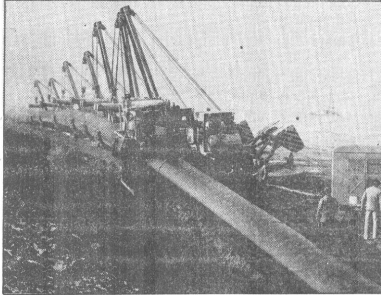
قسمتی از پایپ لاین بزرگی که گاز طبیعی را از اتحاد شوروی به اروپای غربی انتقال میدهد این پایپ لاین بطول ۲۴۳ کیلو متر از سر زمین چکوسلواکی عبور می کند . کارگران این کشور به صورت خستگی ناپذیر تلاش مینمایند تا هر چه زود تر کار بالای این پروژه پایان یابد و به منطقه بو هیان آلمان فدرال برسد .
